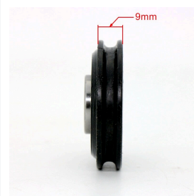
电梯门轮 3201.05.0037P
