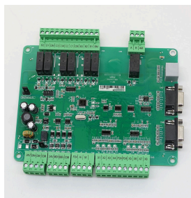
电梯电路板 MCTC-CTB-A
