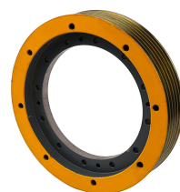
电梯曳引轮 P101041A234-10 400mm 5x8 6x8 Gro?
