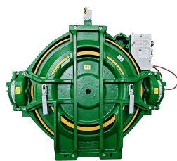
电梯无齿轮曳引机 MX10 NMX11 MX14
