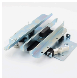
电梯门刀 H1
