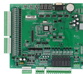
电梯PCB MCTC-MCB-C2
