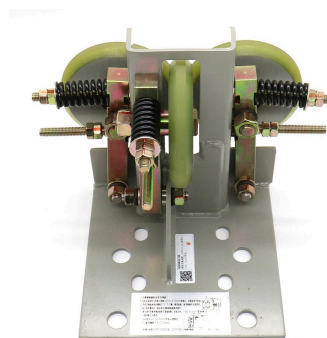
电梯滚轮导靴 C0083111-B
