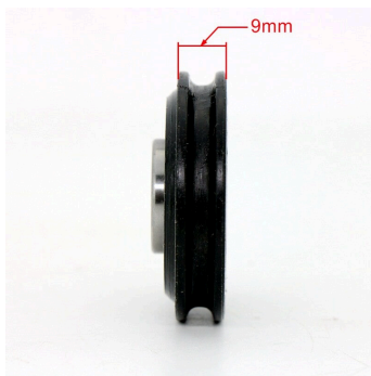
电梯Door Wheel 3201.05.0037P
