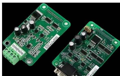
电梯PCB MCTC-PG-E
